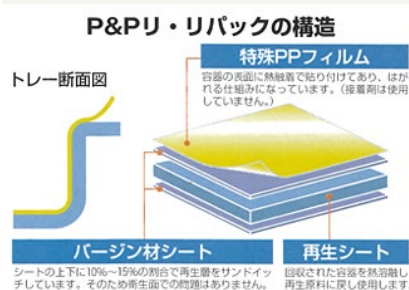
P&Pリ・リパックの構造
